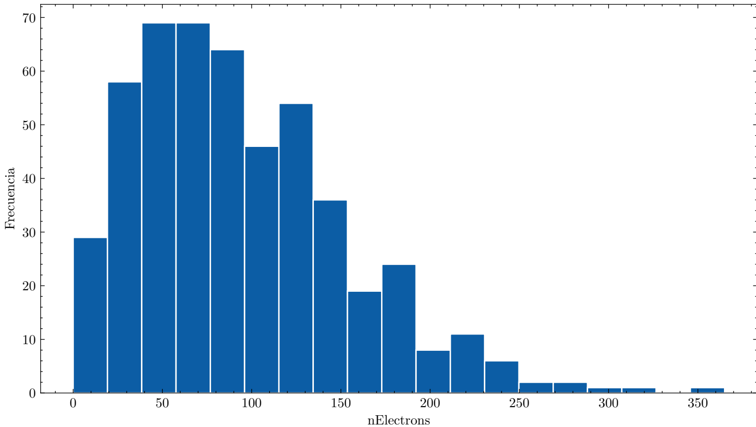
Distribución de nElectrons ar_33.0_cf4_67.0_90.0kVcm_1.000bar_0.0309mm_500npe
