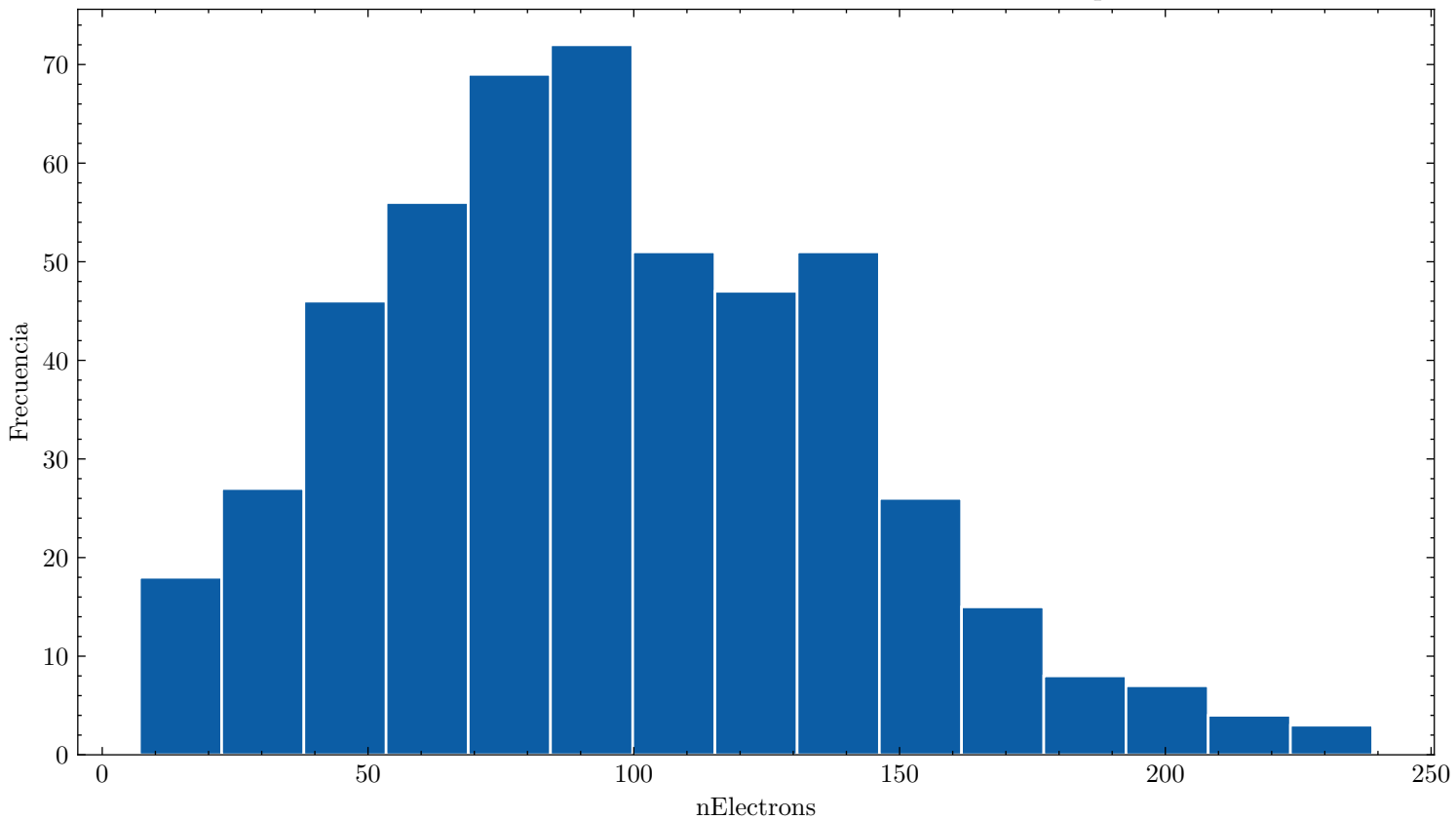
Distribución de nElectrons ar_67.0_cf4_33.0_110.0kVcm_1.000bar_0.0214mm_500npe
