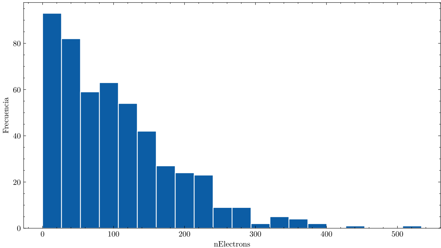
Distribución de nElectrons ar_67.0_cf4_33.0_40.0kVcm_1.000bar_0.1307mm_500npe
