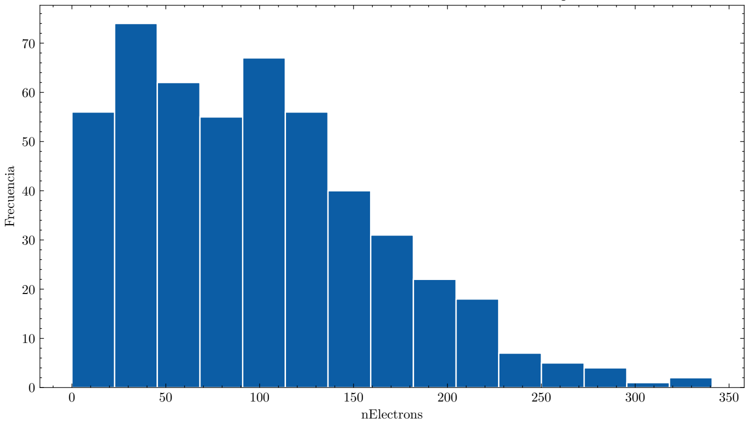
Distribución de nElectrons ar_67.0_cf4_33.0_60.0kVcm_1.000bar_0.0534mm_500npe
