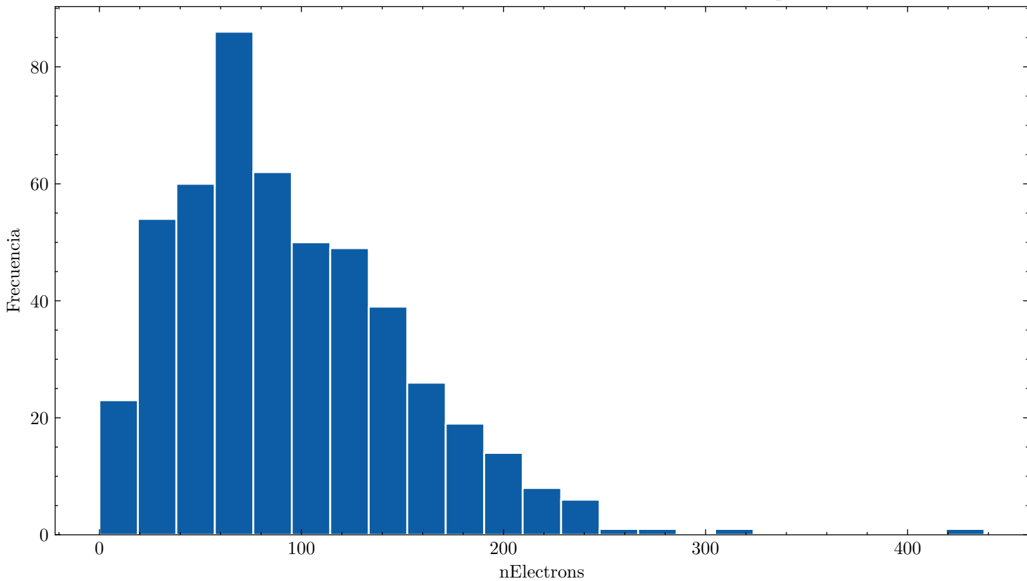
Distribución de nElectrons ar_67.0_cf4_33.0_70.0kVcm_1.000bar_0.0409mm_500npe
