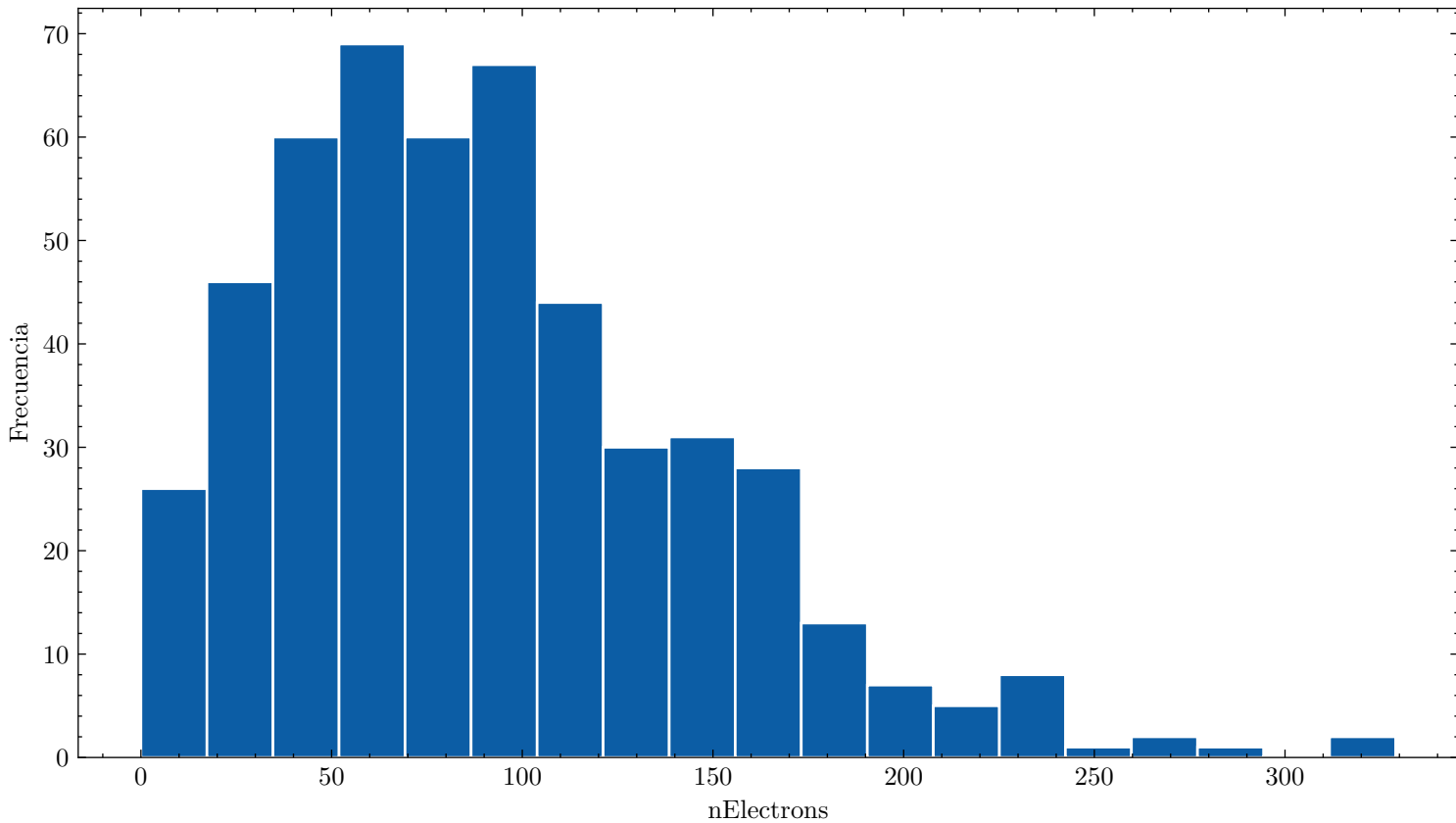
Distribución de nElectrons ar_67.0_cf4_33.0_80.0kVcm_1.000bar_0.0332mm_500npe
