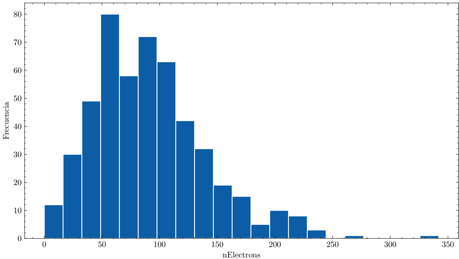
Distribución de nElectrons ar_90.0_cf4_10.0_110.0kVcm_1.000bar_0.0204mm_500npe
