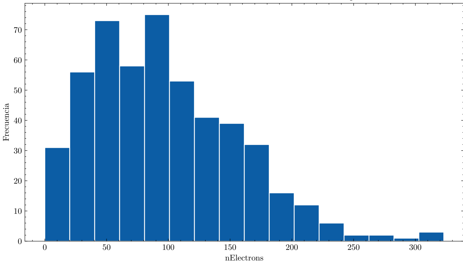
Distribución de nElectrons ar_90.0_cf4_10.0_60.0kVcm_1.000bar_0.0473mm_500npe
