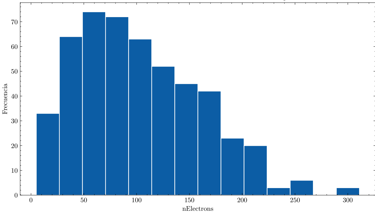
Distribución de nElectrons ar_90.0_cf4_10.0_80.0kVcm_1.000bar_0.0313mm_500npe
