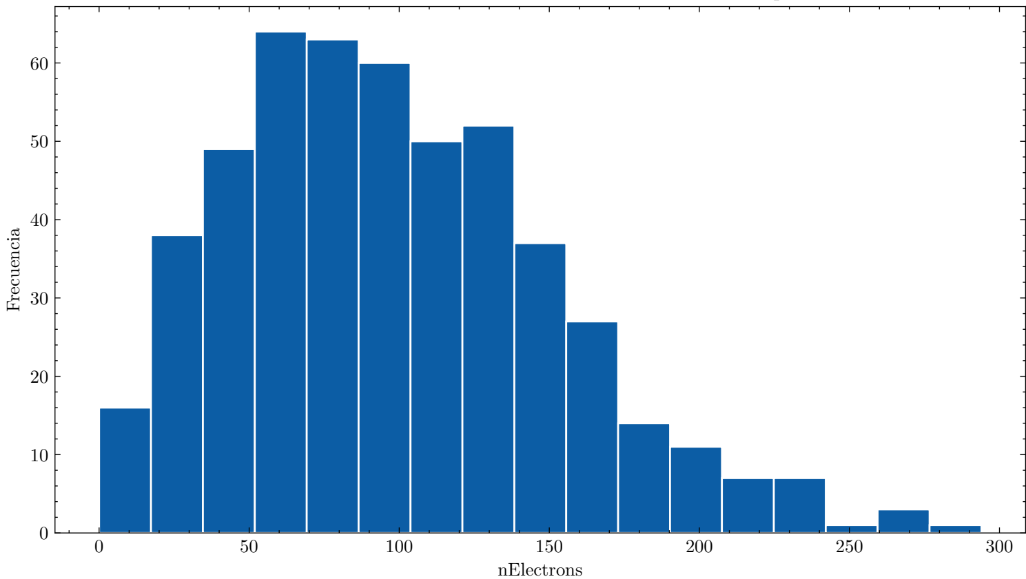
Distribución de nElectrons ar_90.0_cf4_10.0_90.0kVcm_1.000bar_0.0267mm_500npe
