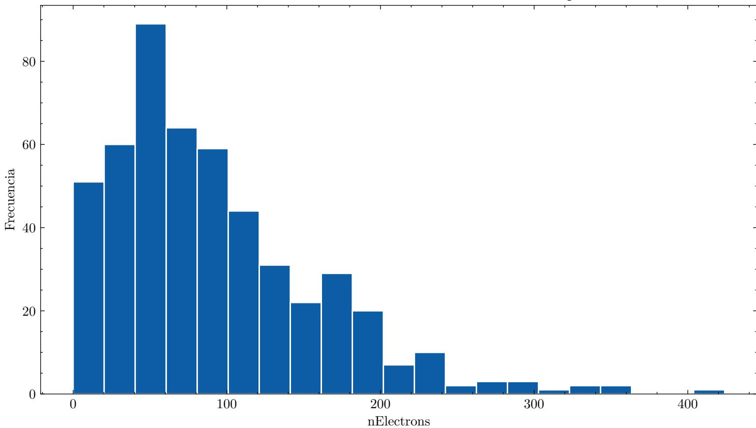
Distribución de nElectrons ar_95.0_cf4_5.0_40.0kVcm_1.000bar_0.0901mm_500npe
