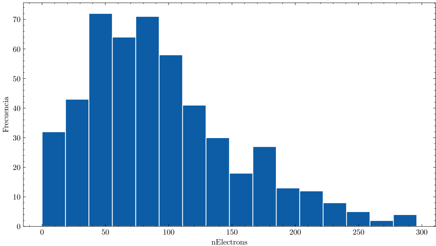
Distribución de nElectrons ar_95.0_cf4_5.0_60.0kVcm_1.000bar_0.0461mm_500npe
