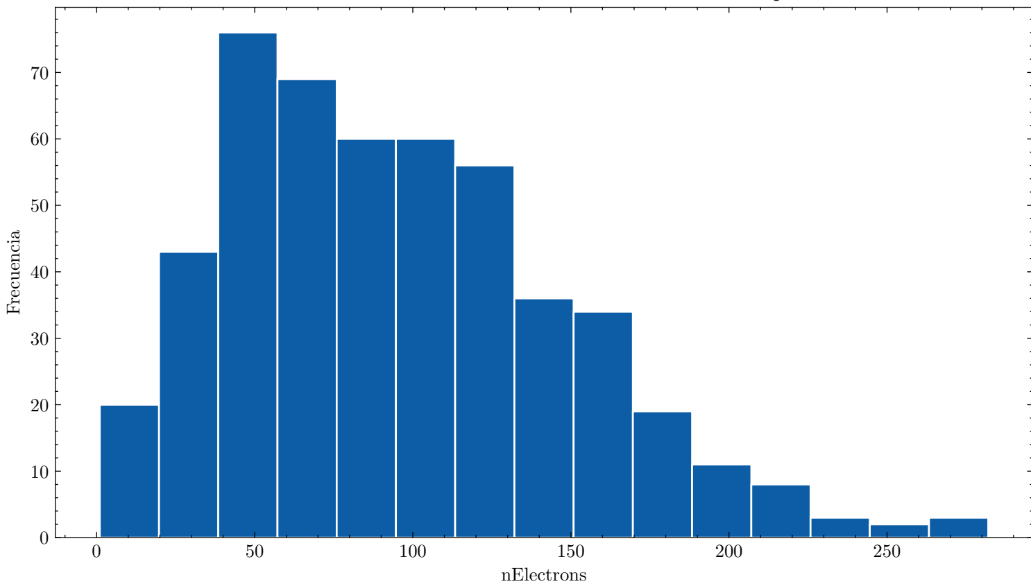
Distribución de nElectrons ar_95.0_cf4_5.0_80.0kVcm_1.000bar_0.0307mm_500npe
