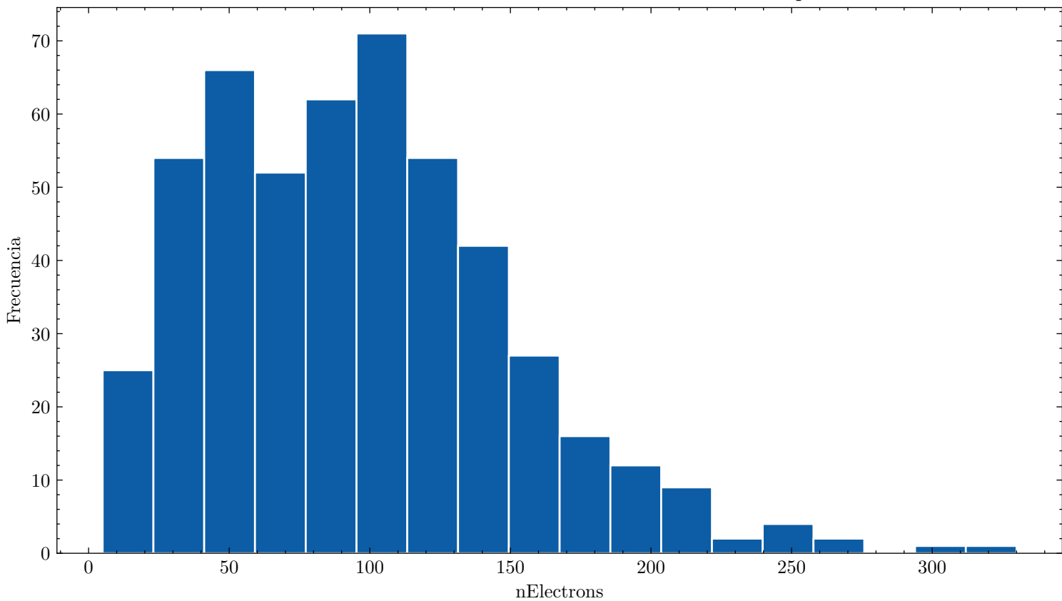
Distribución de nElectrons ar_95.0_cf4_5.0_90.0kVcm_1.000bar_0.0262mm_500npe
