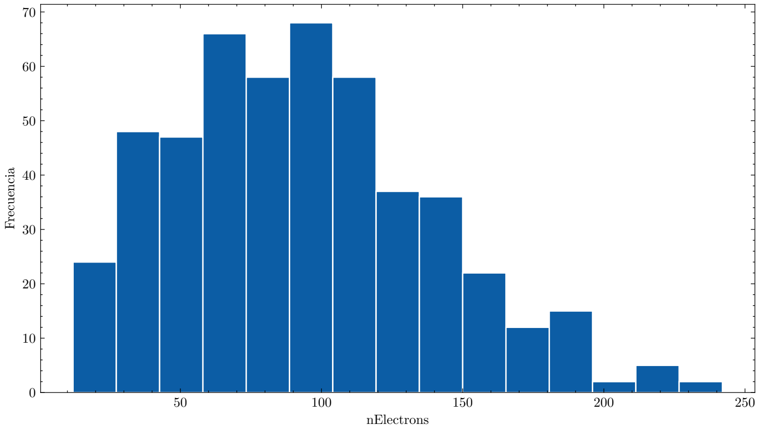
Distribución de nElectrons ar_99.0_cf4_1.0_110.0kVcm_1.000bar_0.0201mm_500npe
