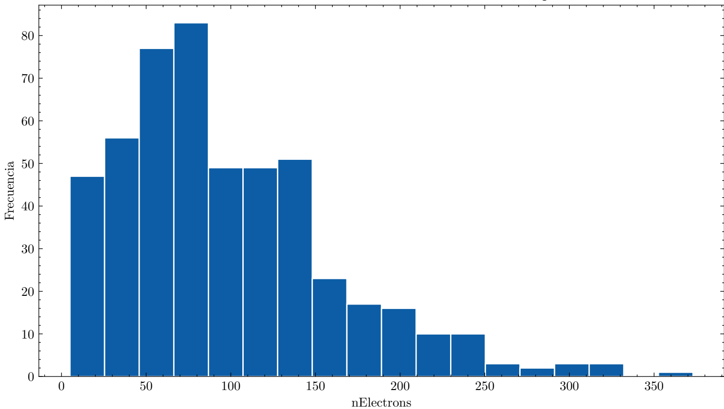
Distribución de nElectrons ar_99.0_cf4_1.0_60.0kVcm_1.000bar_0.0452mm_500npe
