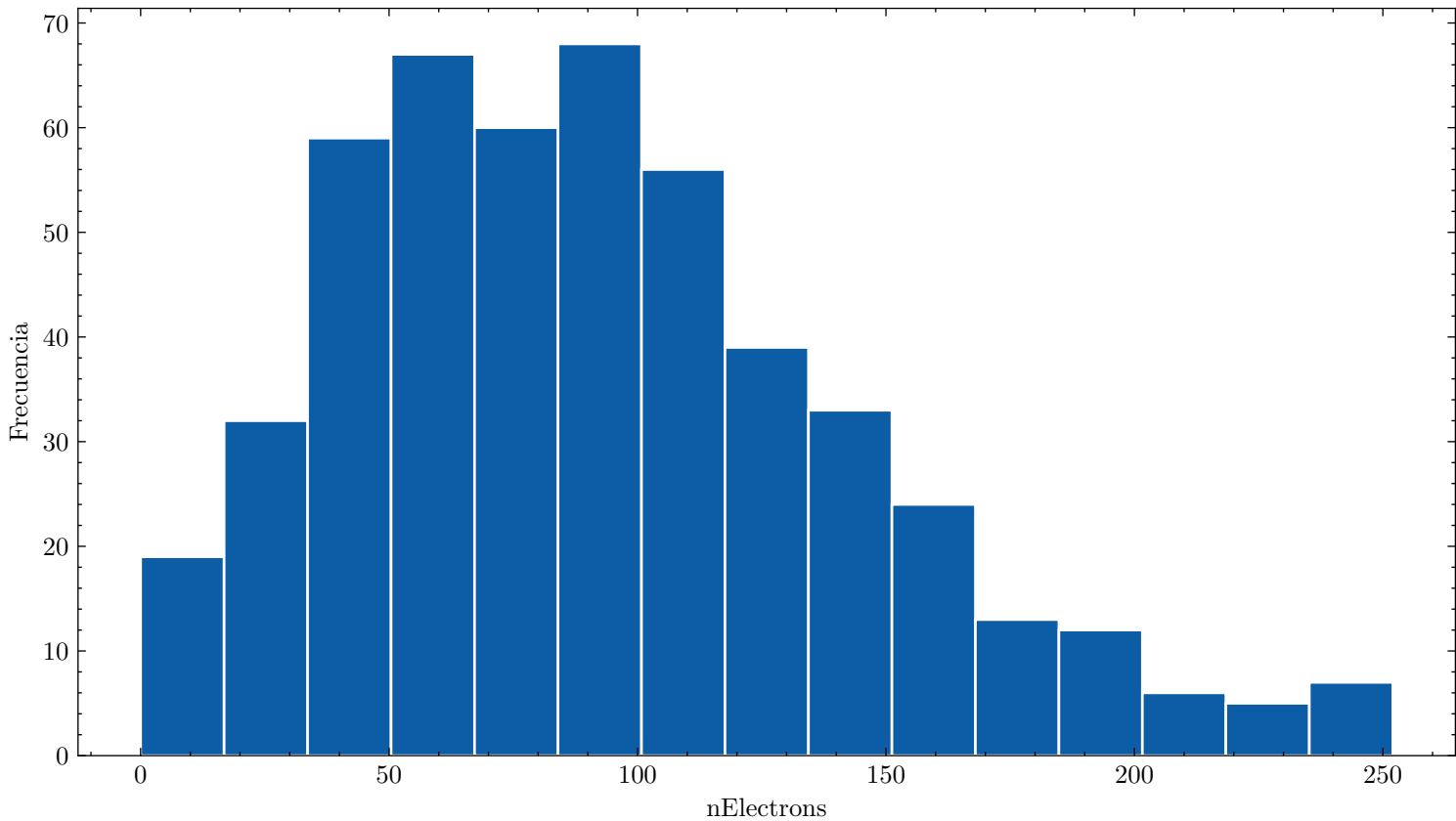
Distribución de nElectrons cf4_100.0_ar_0.0_110.0kVcm_1.000bar_0.0250mm_500npe
