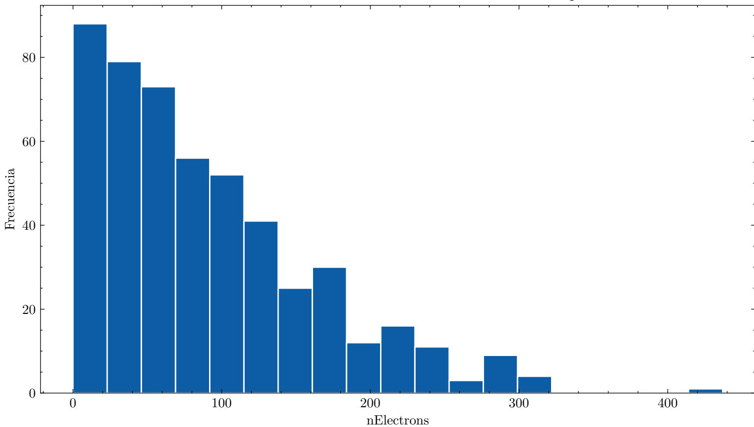
Distribución de nElectrons cf4_100.0_ar_0.0_60.0kVcm_1.000bar_0.0813mm_500npe
