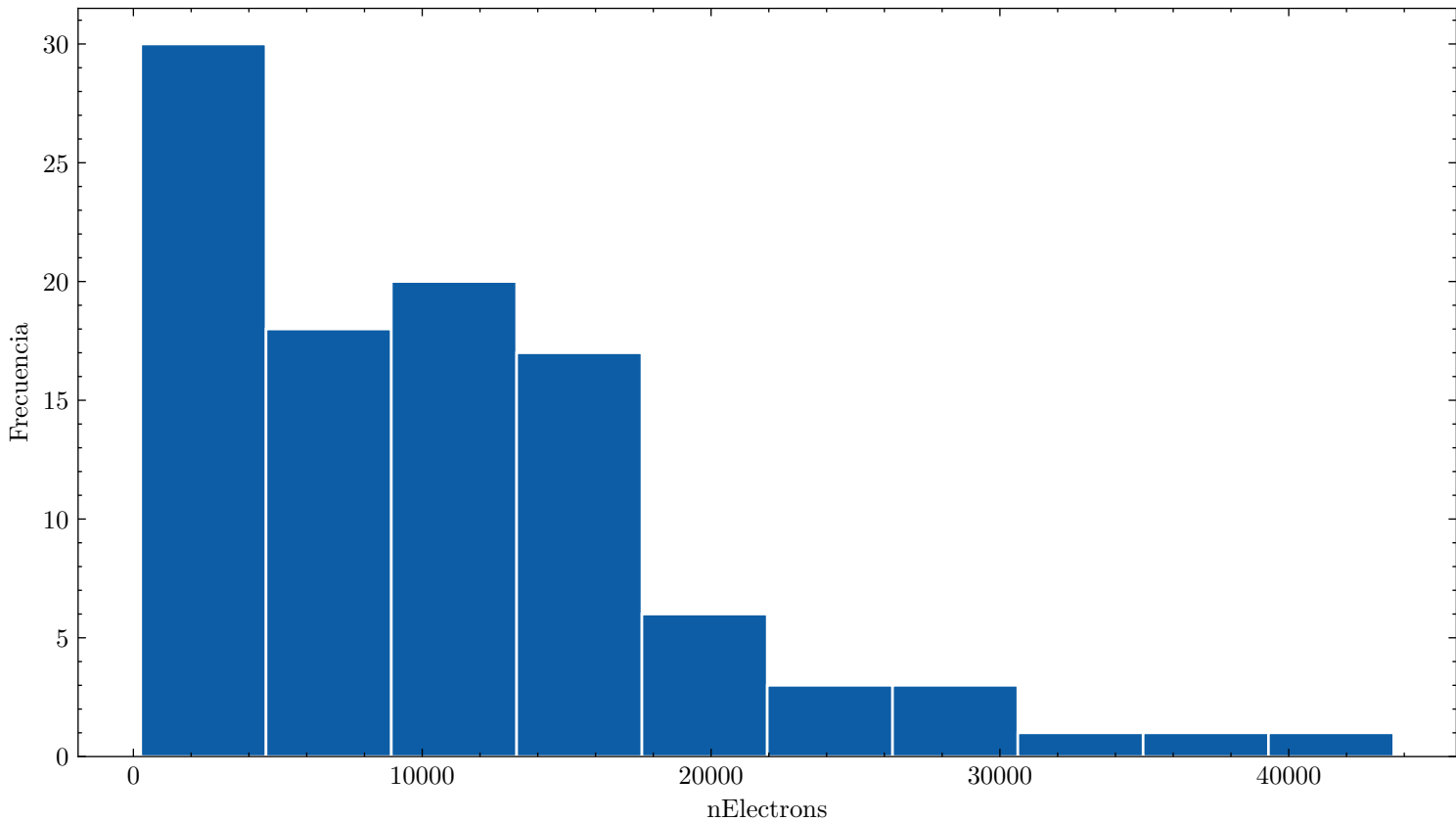
Distribución de nElectrons ar_0.0_n2_100.0_80.0kVcm_1.000bar_0.2124mm_100npe
