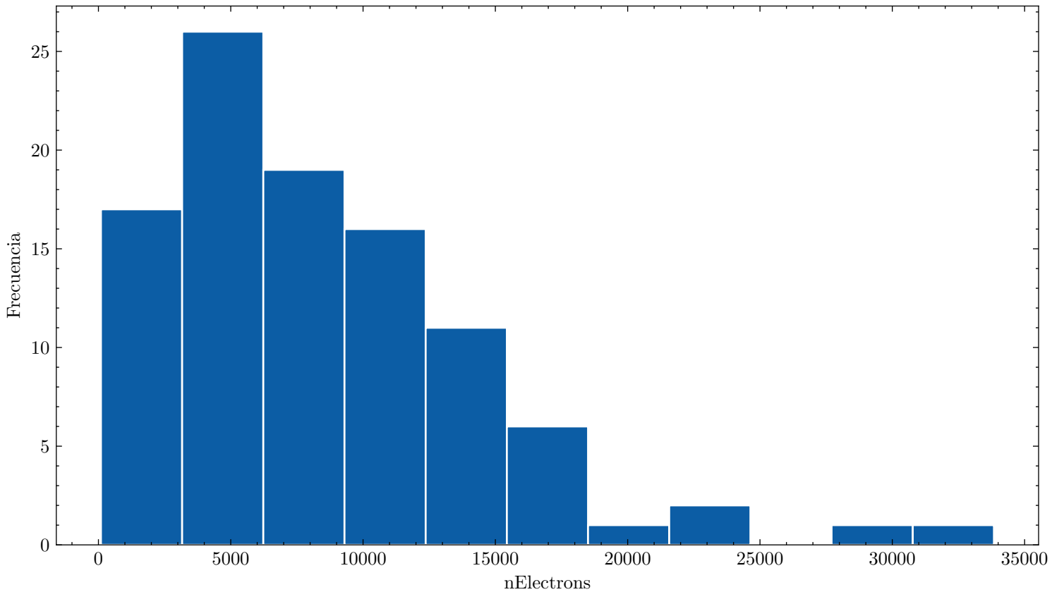
Distribución de nElectrons ar_0.0_n2_100.0_90.0kVcm_1.000bar_0.1587mm_100npe
