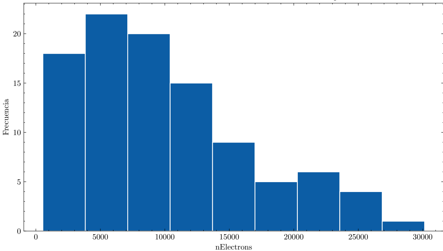
Distribución de nElectrons ar_100.0_n2_0.0_60.0kVcm_1.000bar_0.0901mm_100npe
