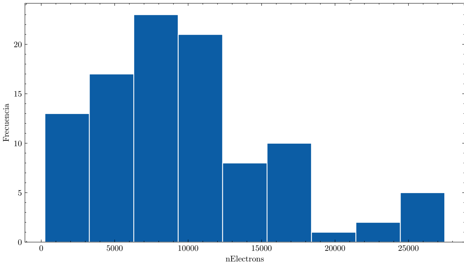
Distribución de nElectrons ar_100.0_n2_0.0_70.0kVcm_1.000bar_0.0722mm_100npe
