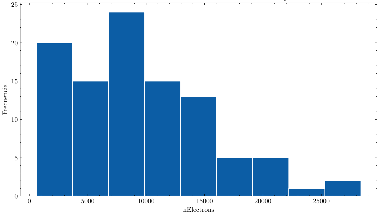
Distribución de nElectrons ar_100.0_n2_0.0_80.0kVcm_1.000bar_0.0602mm_100npe
