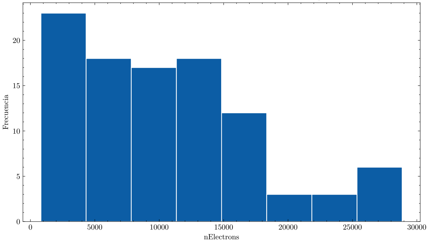
Distribución de nElectrons ar_90.0_n2_10.0_60.0kVcm_1.000bar_0.1071mm_100npe
