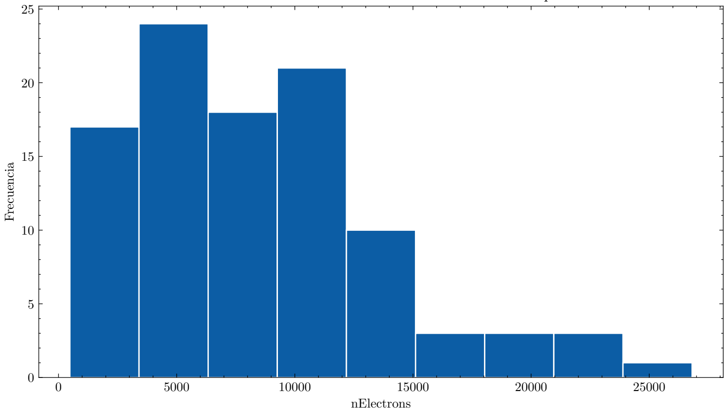
Distribución de nElectrons ar_90.0_n2_10.0_90.0kVcm_1.000bar_0.0572mm_100npe
