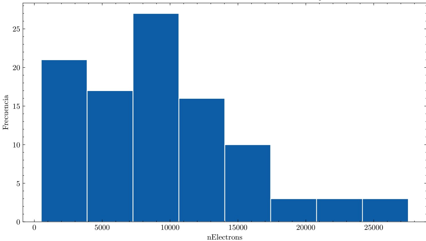
Distribución de nElectrons ar_99.0_n2_1.0_60.0kVcm_1.000bar_0.0914mm_100npe
