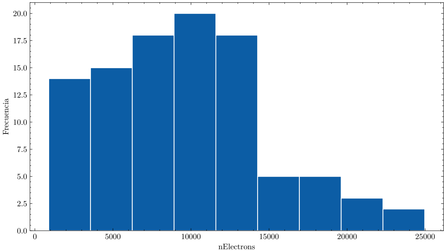
Distribución de nElectrons ar_99.0_n2_1.0_80.0kVcm_1.000bar_0.0608mm_100npe
