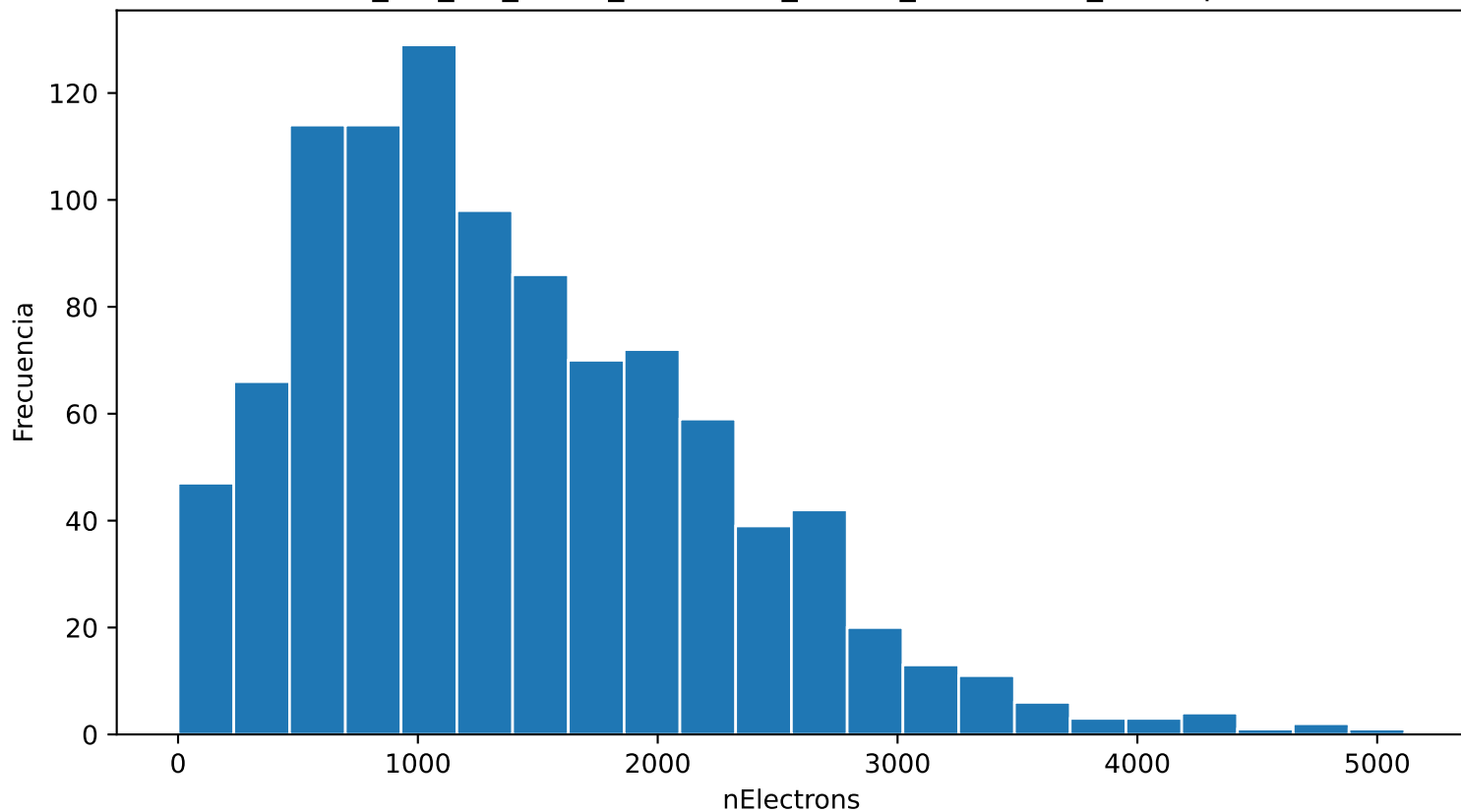
Distribución de nElectrons ar_0.0_cf4_100.0_95.0kVcm_1.0bar_0.0500mm_1000npe
