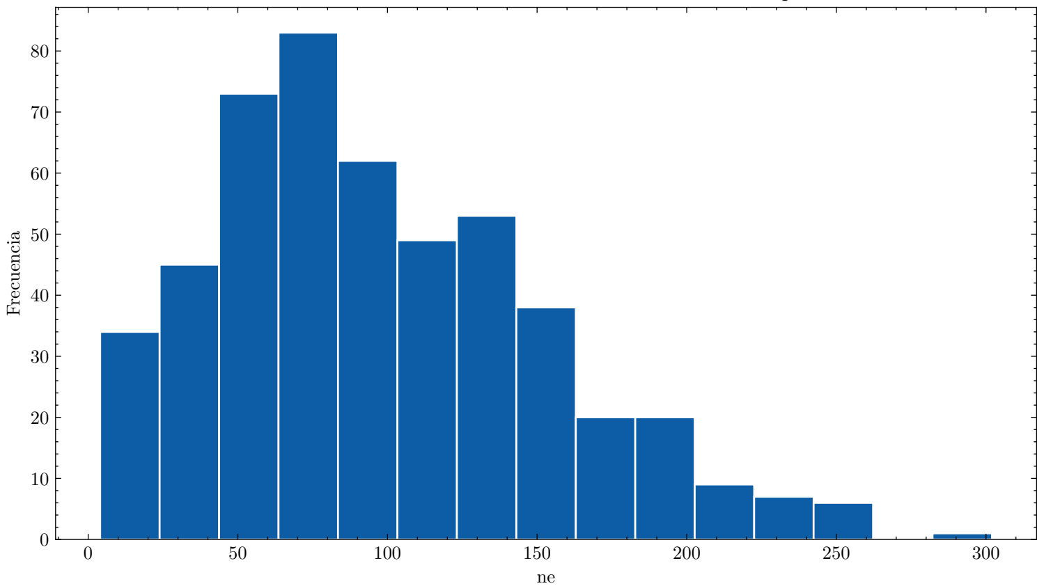
Distribución de ne ar_100.0_cf4_0.0_80.0kVcm_1.000bar_0.0302mm_500npe
