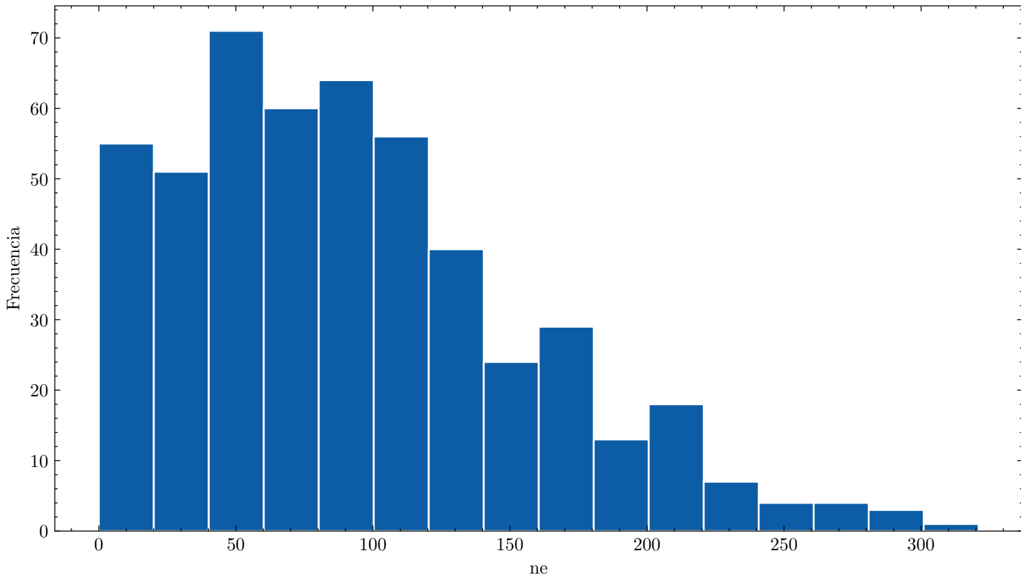
Distribución de ne ar_33.0_cf4_67.0-70.0kVcm_1.000bar_0.0475mm_500npe
