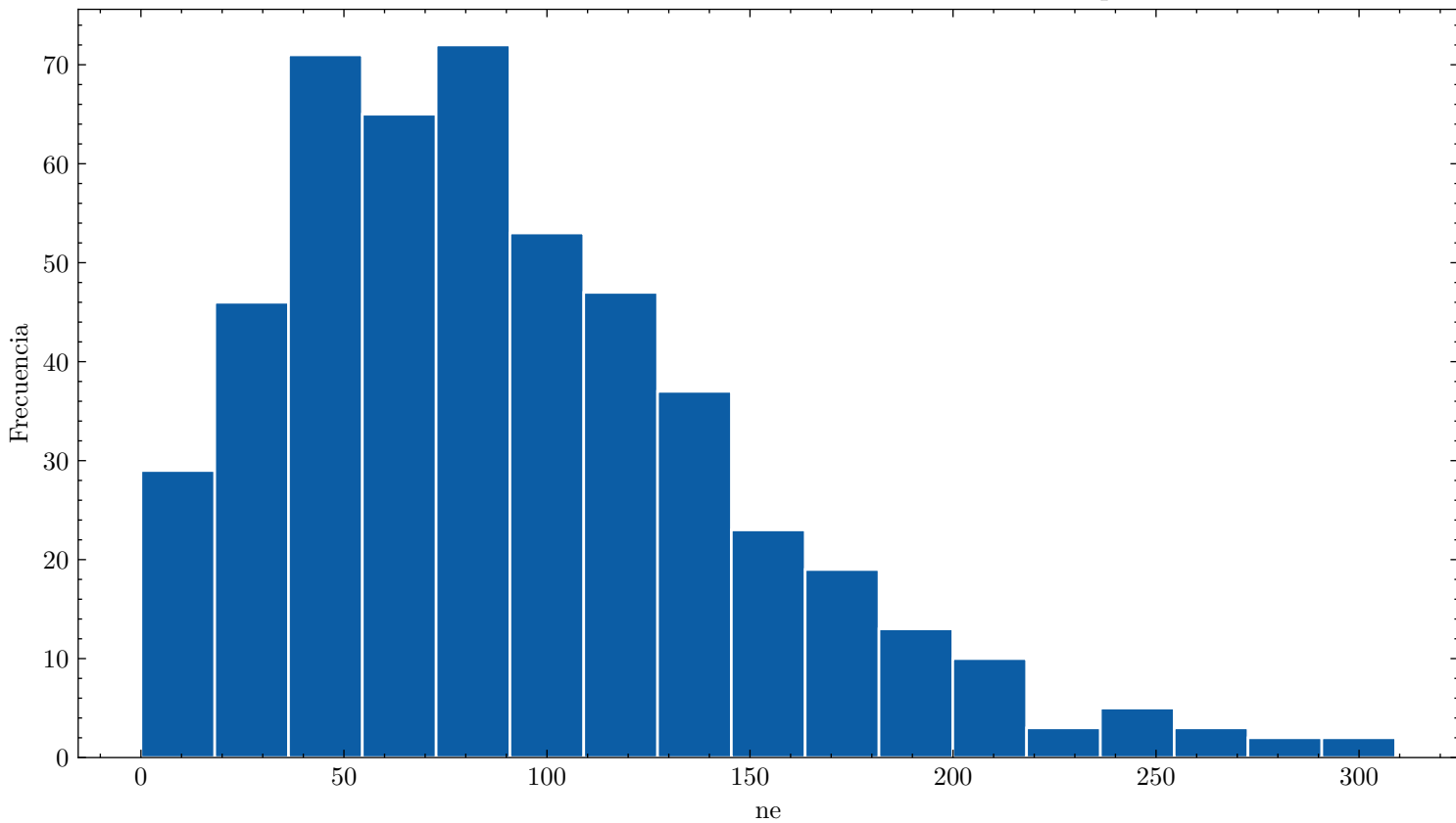
Distribución de ne ar_33.0_cf4_67.0_80.0kVcm_1.000bar_0.0374mm_500npe
