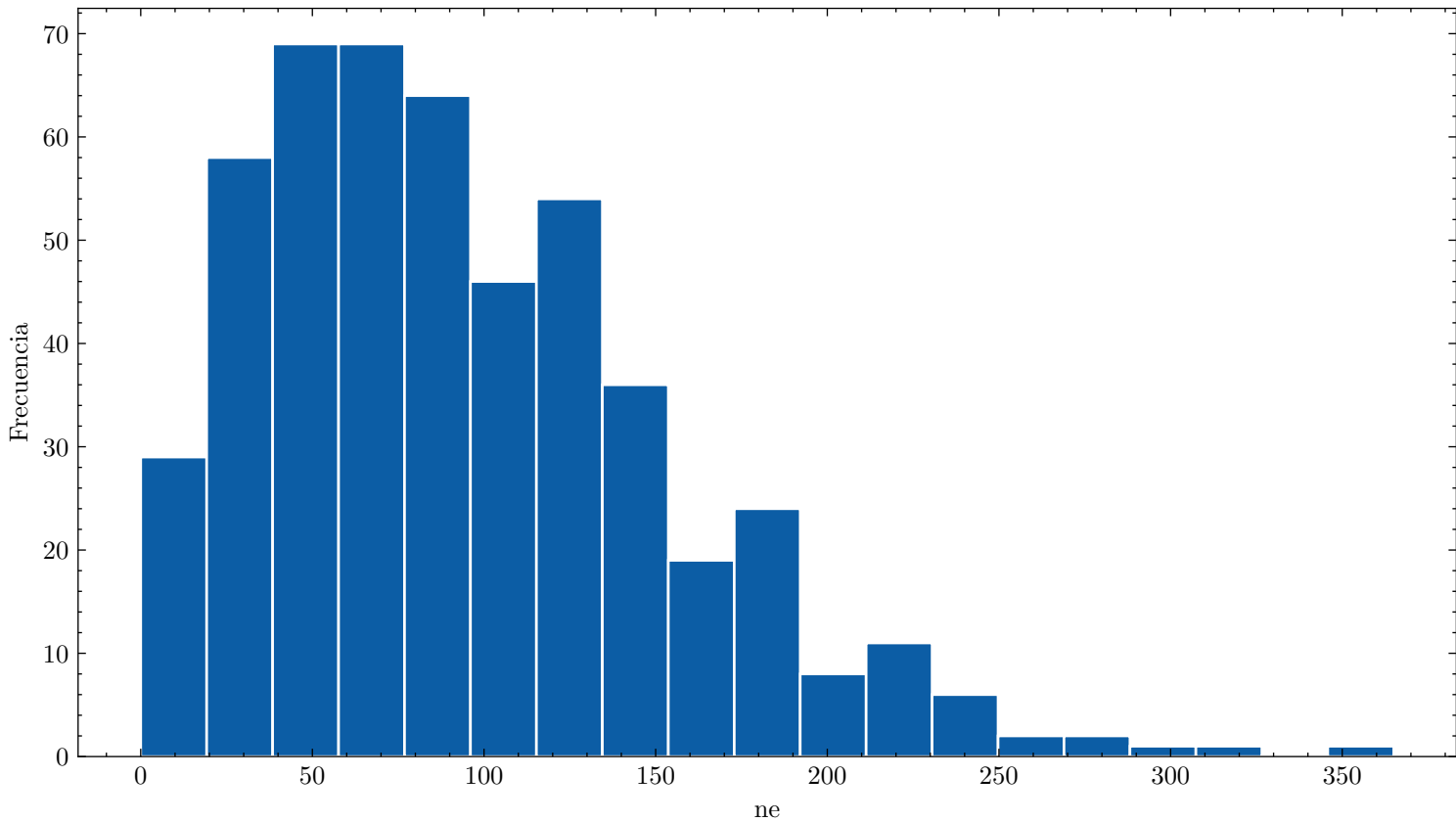
Distribución de ne ar_33.0_cf4_67.0_90.0kVcm_1.000bar_0.0309mm_500npe
