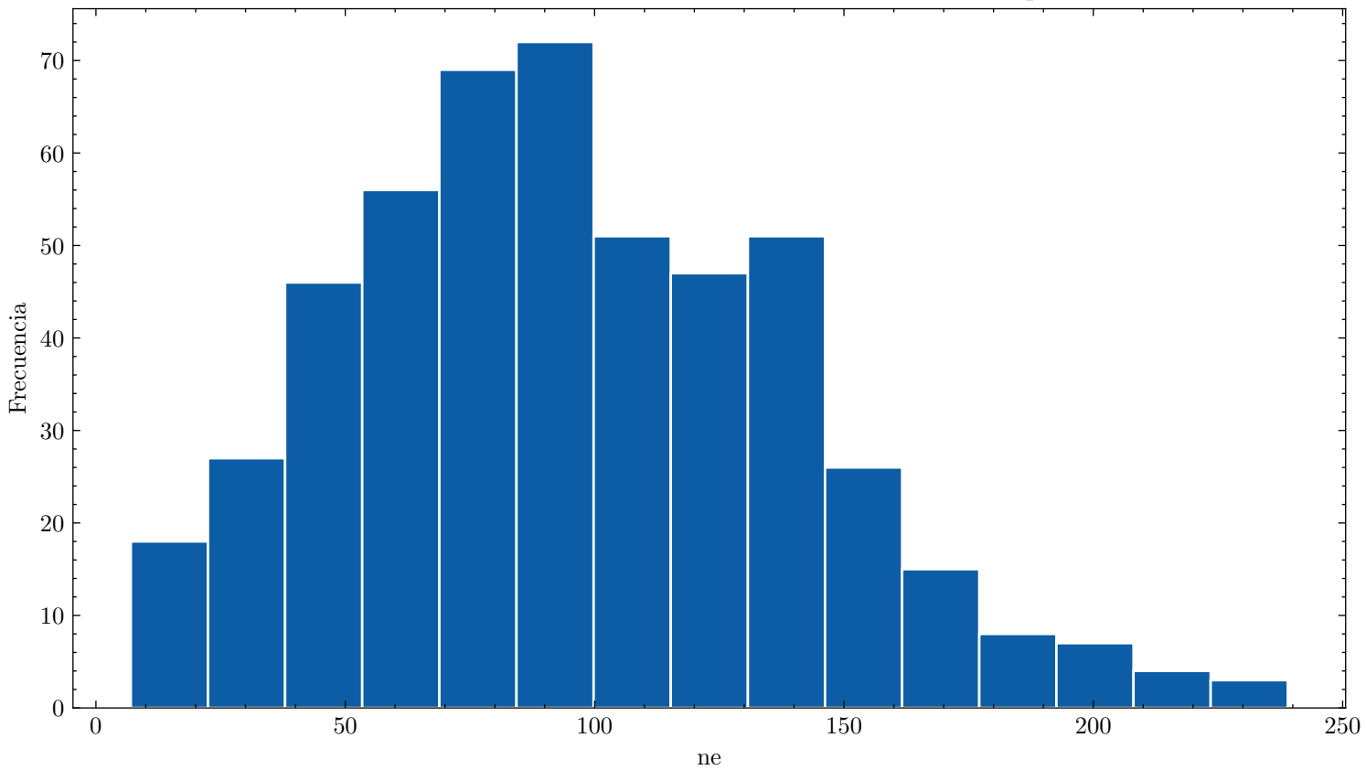
Distribución de ne ar_67.0_cf4_33.0_110.0kVcm_1.000bar_0.0214mm_500npe
