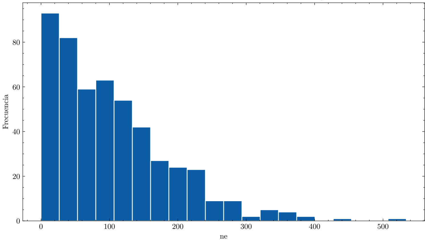
Distribución de ne ar_67.0_cf4_33.0_40.0kVcm_1.000bar_0.1307mm_500npe
