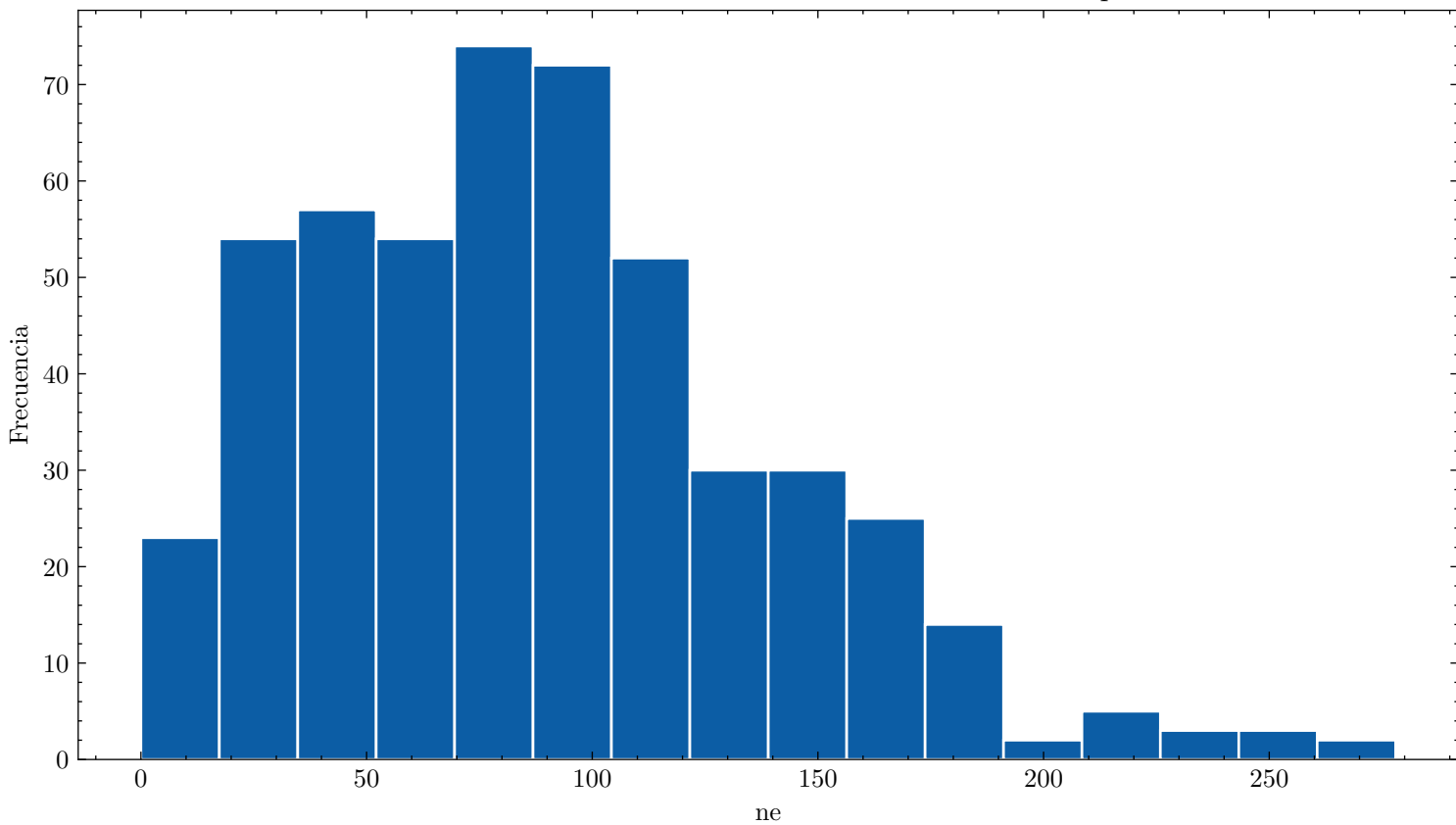
Distribución de ne ar_67.0_cf4_33.0_90.0kVcm_1.000bar_0.0280mm_500npe
