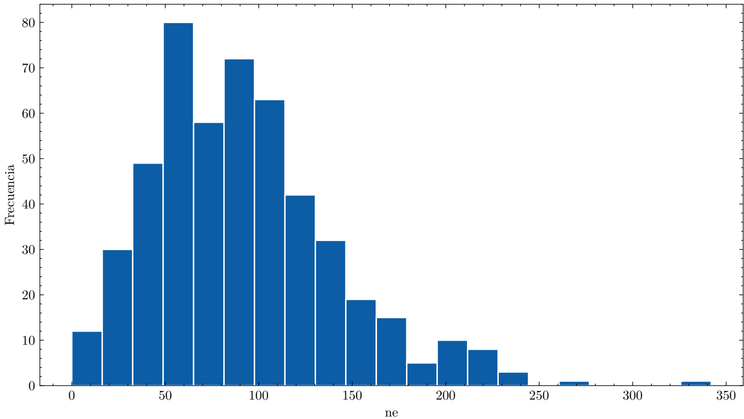
Distribución de ne ar_90.0_cf4_10.0_110.0kVcm_1.000bar_0.0204mm_500npe
