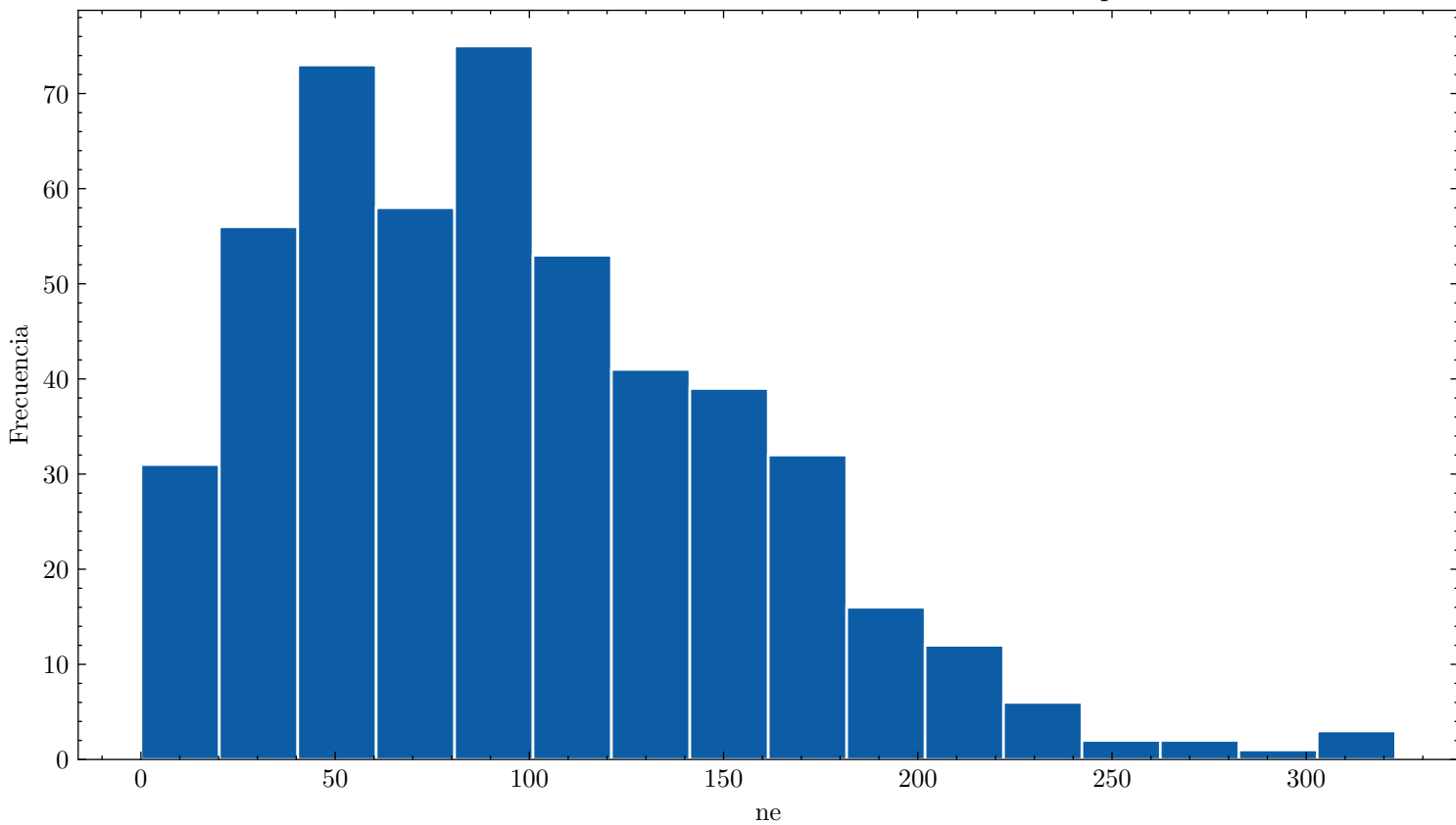
Distribución de ne ar_90.0_cf4_10.0_60.0kVcm_1.000bar_0.0473mm_500npe
