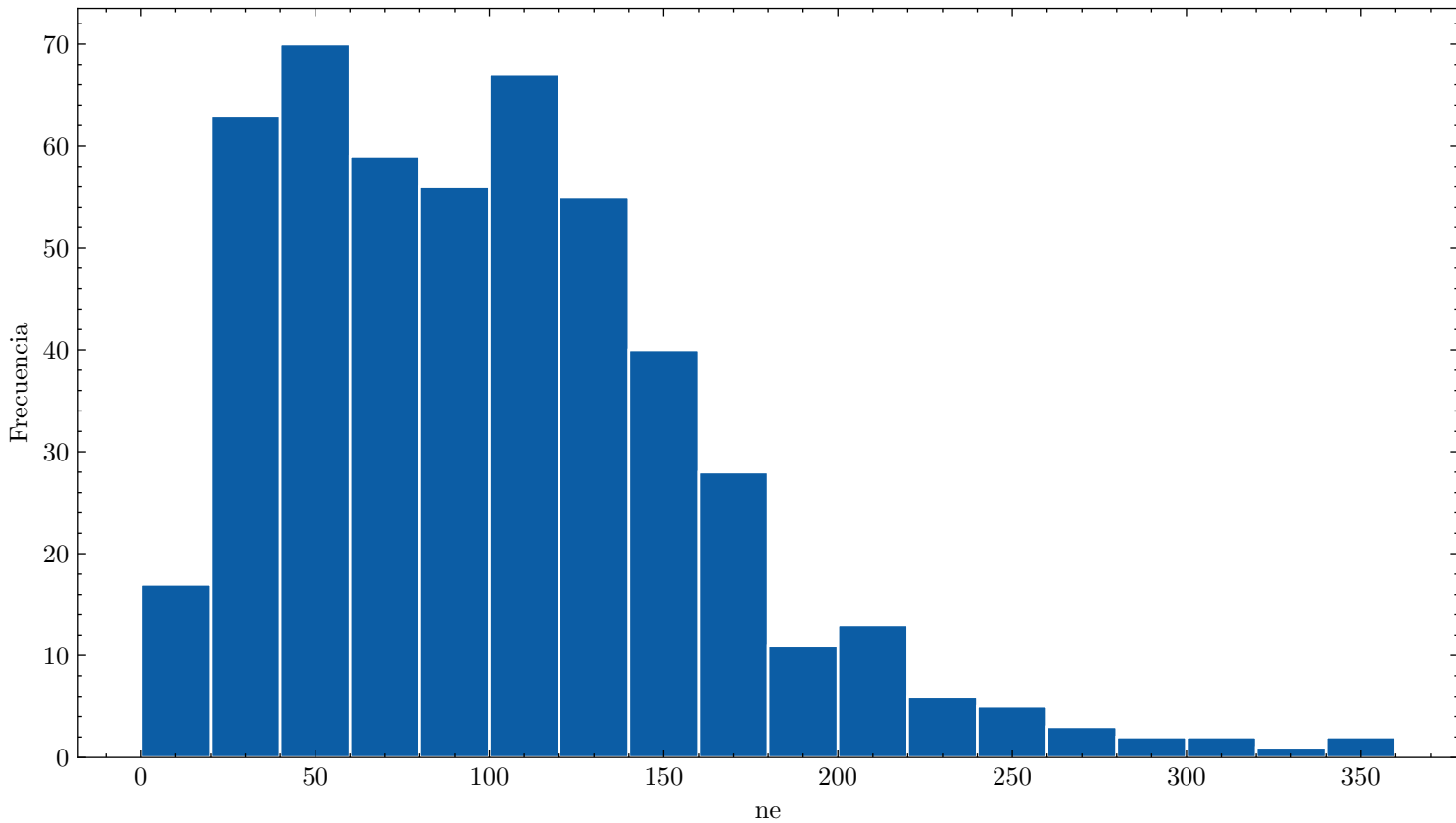
Distribución de ne ar_90.0_cf4_10.0_70.0kVcm_1.000bar_0.0378mm_500npe
