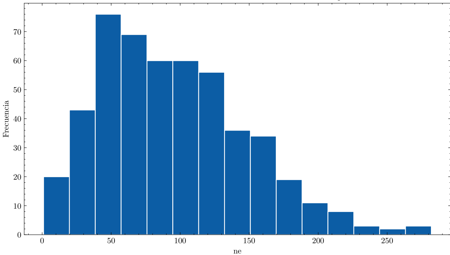
Distribución de ne ar_95.0_cf4_5.0_80.0kVcm_1.000bar_0.0307mm_500npe
