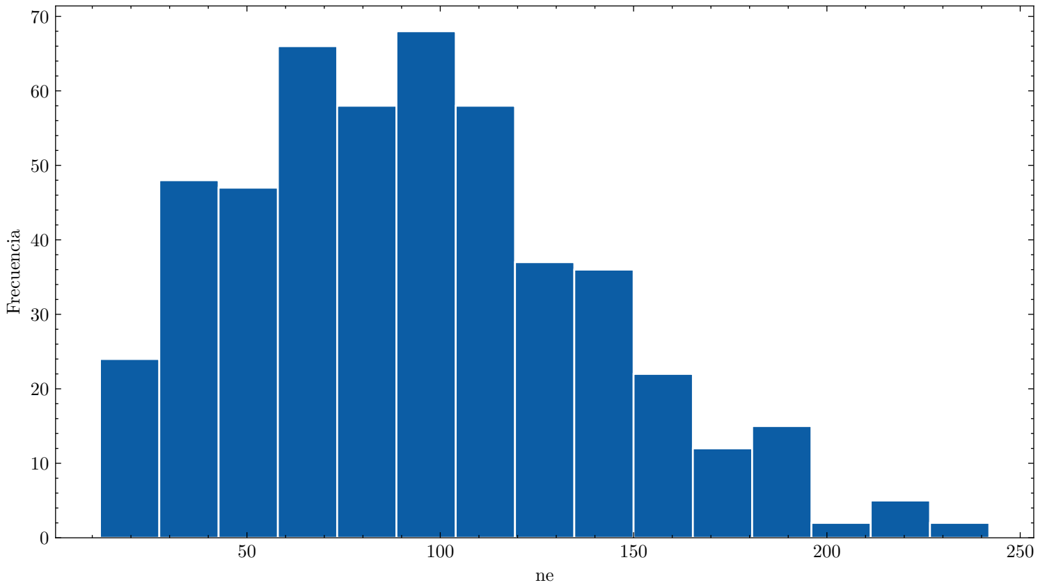
Distribución de ne ar_99.0_cf4_1.0_110.0kVcm_1.000bar_0.0201mm_500npe
