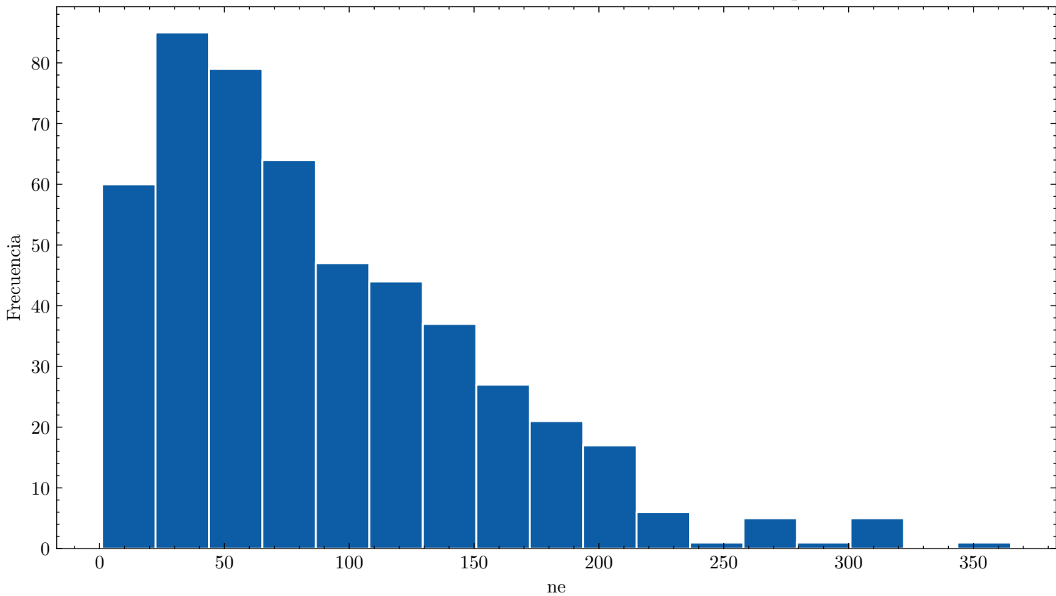
Distribución de ne ar_99.0_cf4_1.0_40.0kVcm_1.000bar_0.0872mm_500npe
