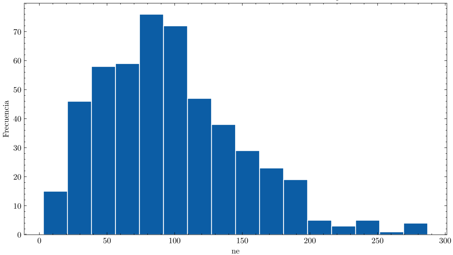
Distribución de ne ar_99.0_cf4_1.0_90.0kVcm_1.000bar_0.0259mm_500npe
