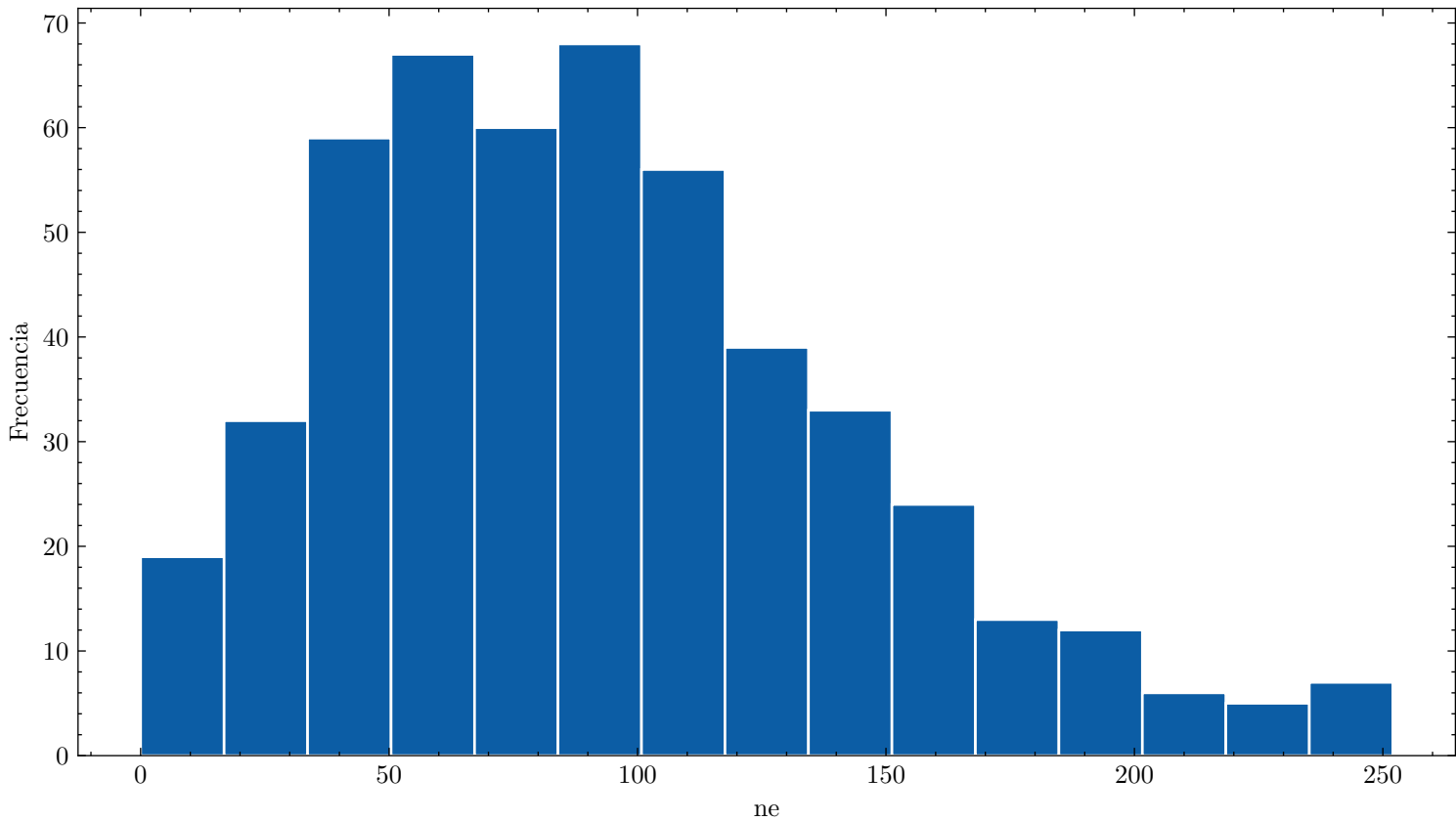
Distribución de ne cf4_100.0_ar_0.0_110.0kVcm_1.000bar_0.0250mm_500npe
