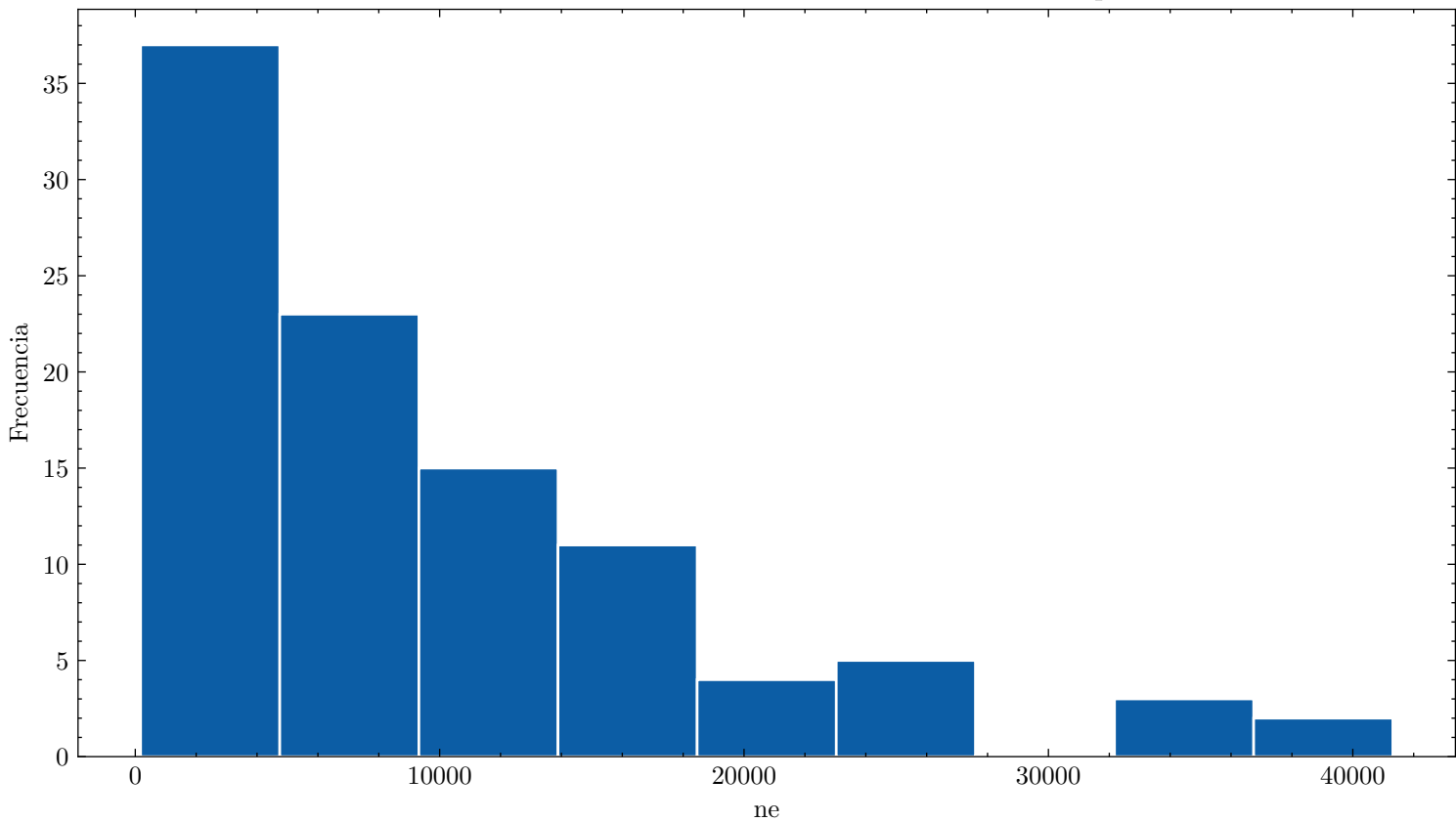
Distribución de ne ar_0.0_n2_100.0_70.0kVcm_1.000bar_0.3030mm_100npe
