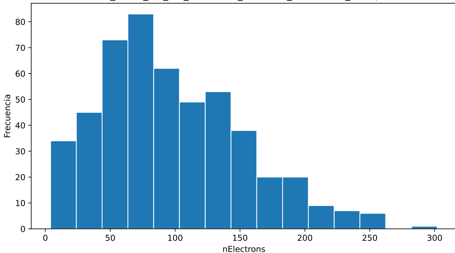
Distribución de nElectrons ar_100.0_cf4_0.0_80.0kVcm_1.000bar_0.0302mm_500npe
