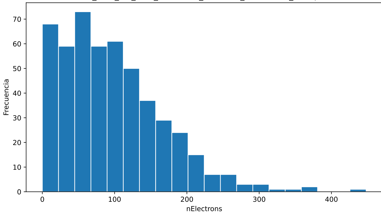
Distribución de nElectrons ar_33.0_cf4_67.0_60.0kVcm_1.000bar_0.0653mm_500npe
