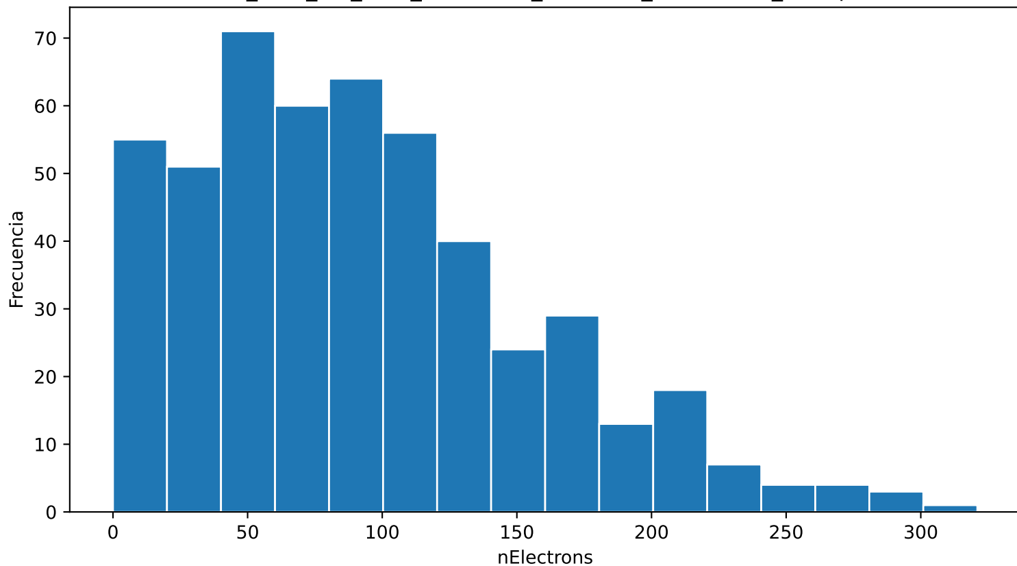
Distribución de nElectrons ar_33.0_cf4_67.0_70.0kVcm_1.000bar_0.0475mm_500npe
