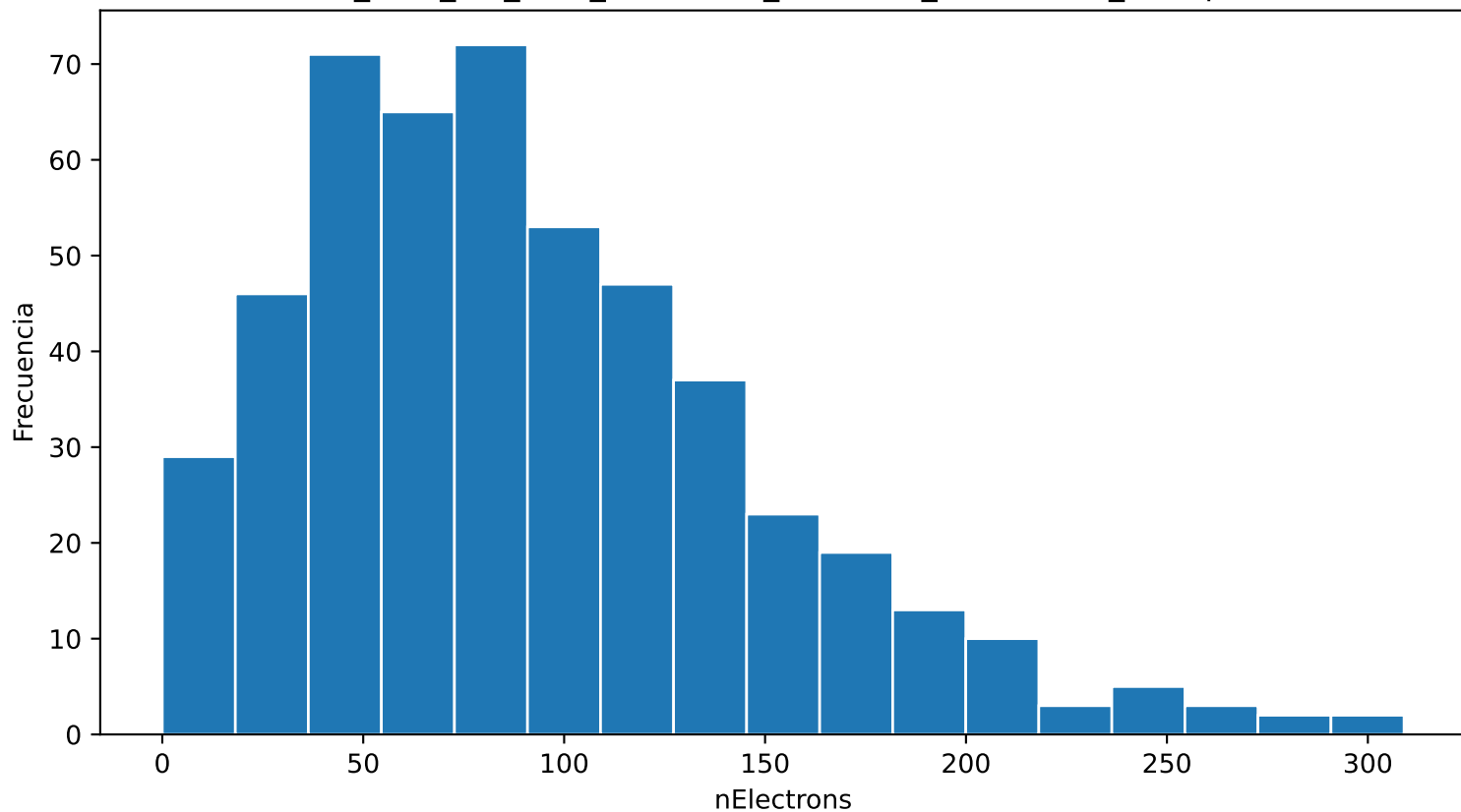
Distribución de nElectrons ar_33.0_cf4_67.0_80.0kVcm_1.000bar_0.0374mm_500npe
