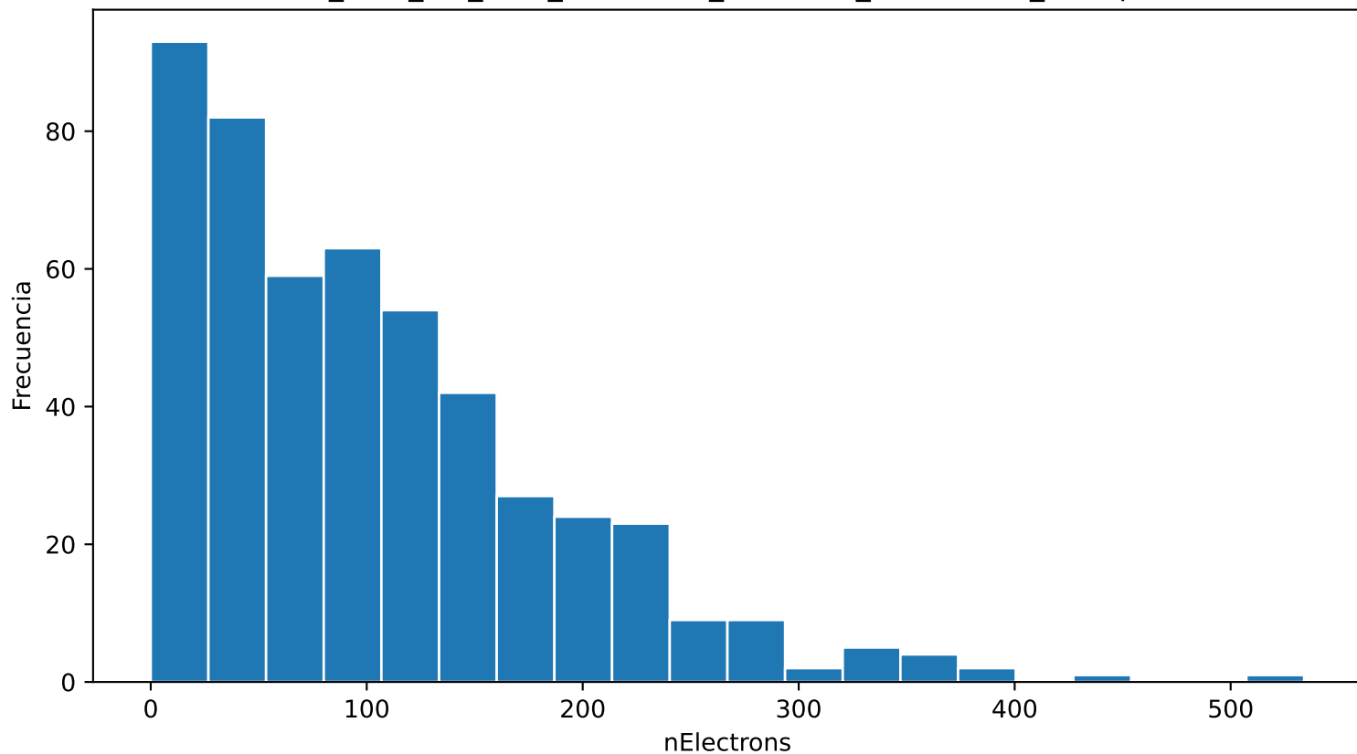
Distribución de nElectrons ar_67.0_cf4_33.0_40.0kVcm_1.000bar_0.1307mm_500npe
