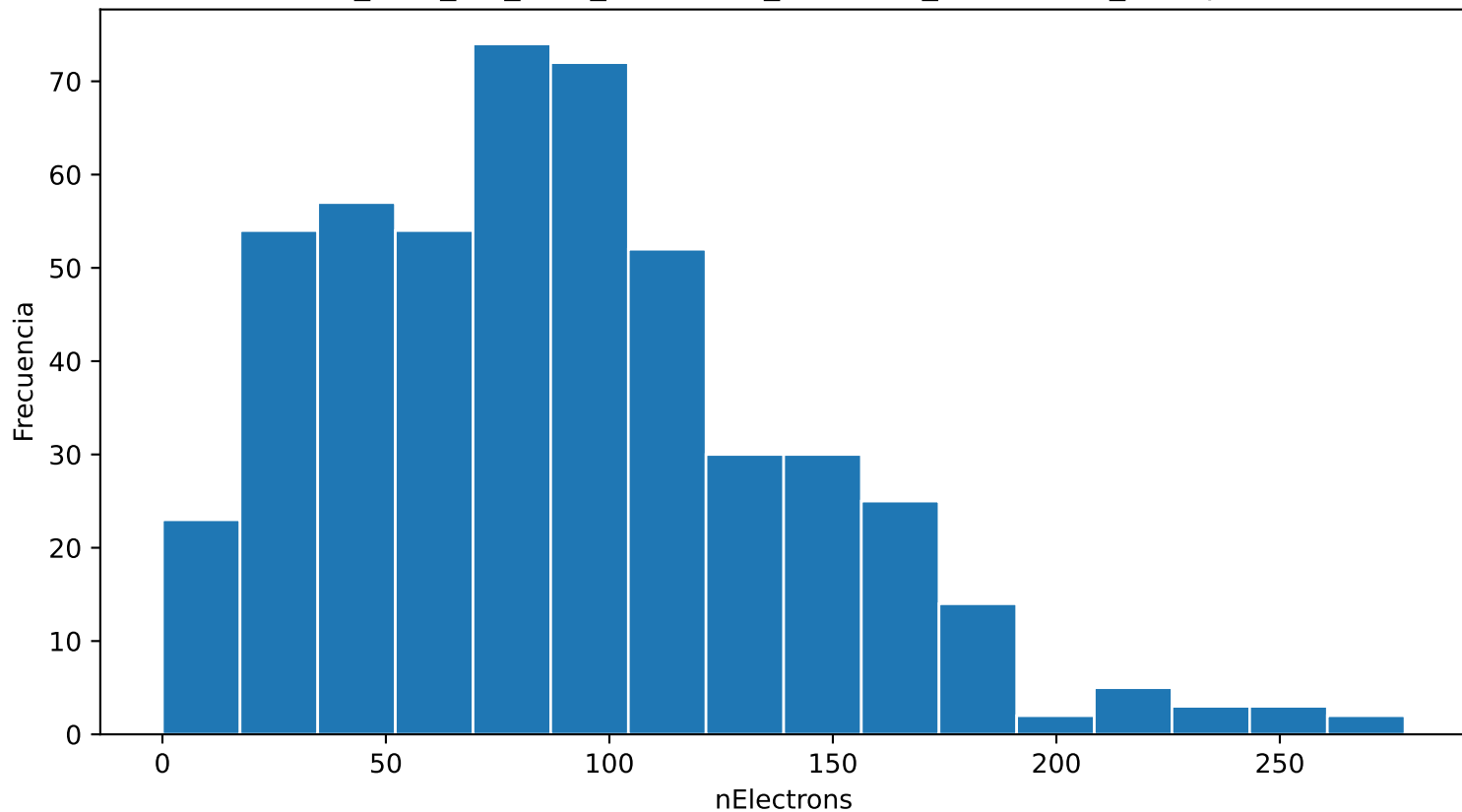
Distribución de nElectrons ar_67.0_cf4_33.0_90.0kVcm_1.000bar_0.0280mm_500npe
